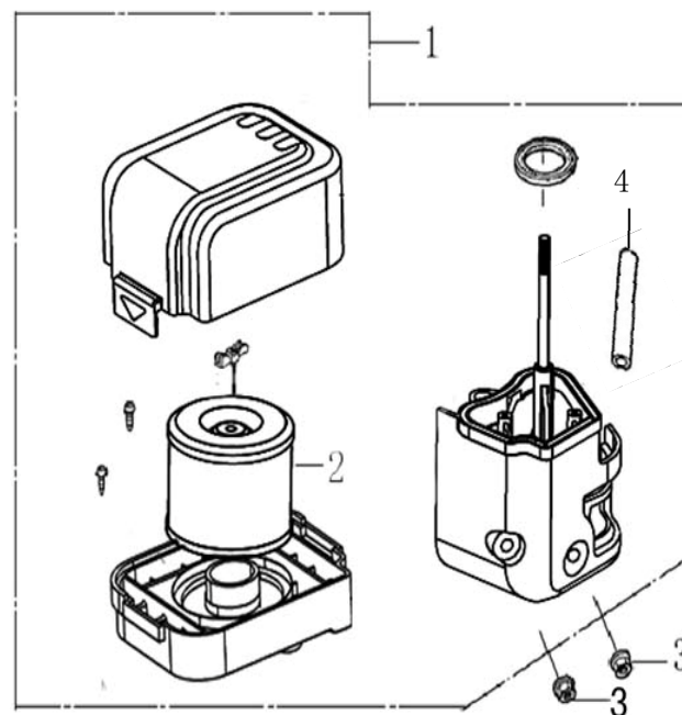
Vzduchový filtr
