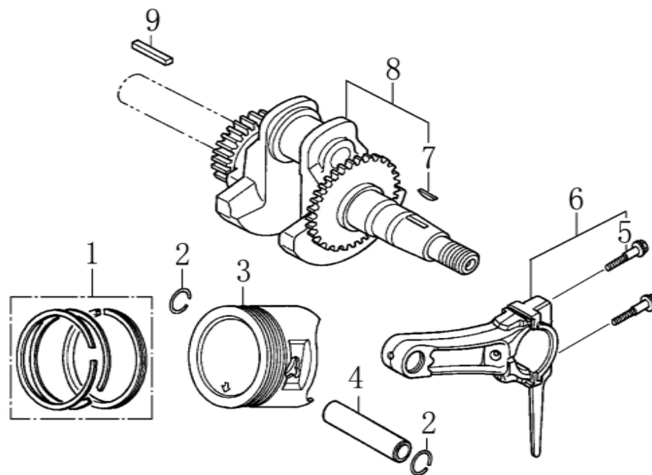
Kliková hřídel, Píst, Ojnice
