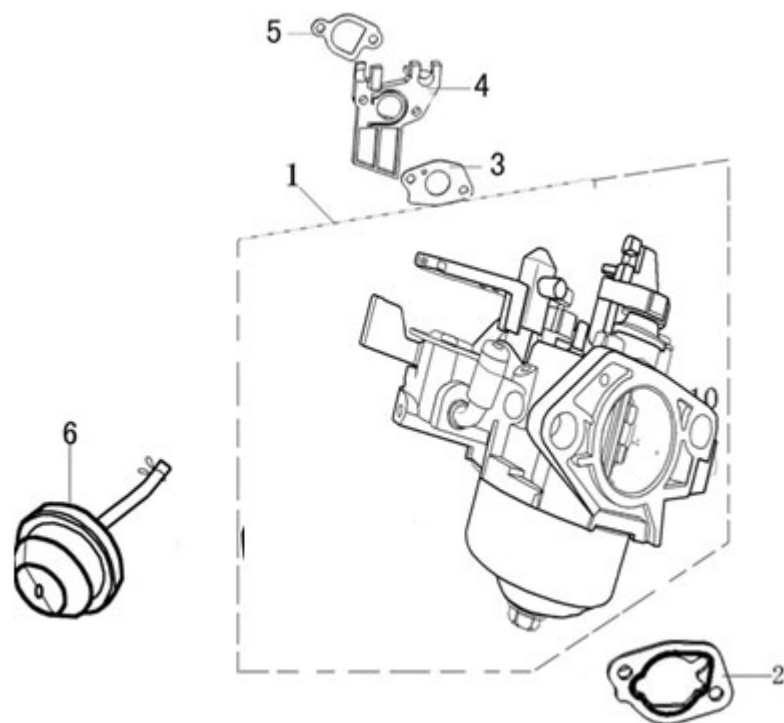
Karburátor
