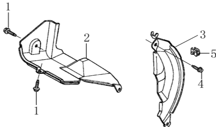
Kryty
