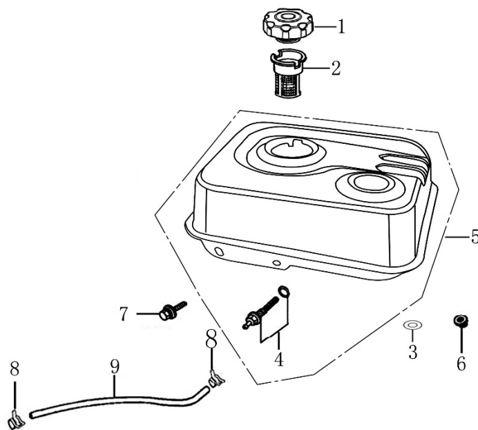
Palivová nádrž
