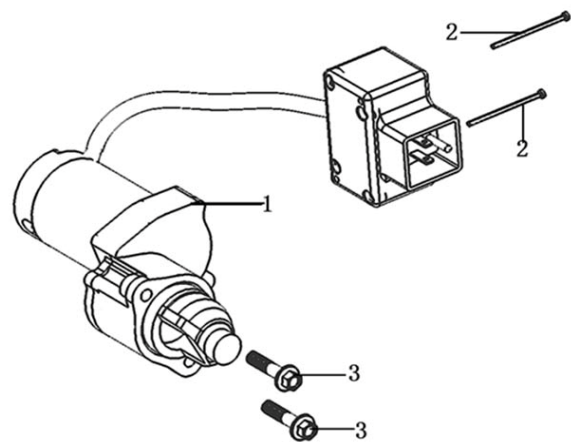
Elektrický startér
